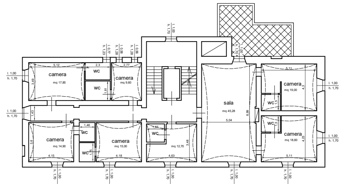
PIANO SECONDO
