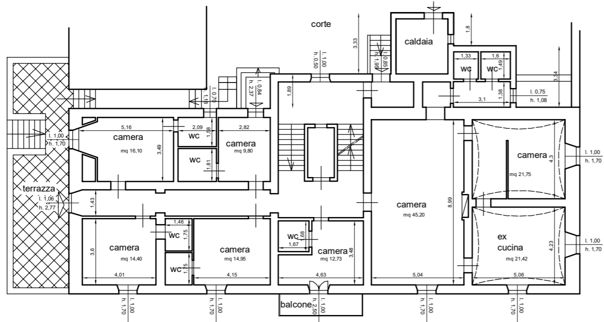
PIANO PRIMO
